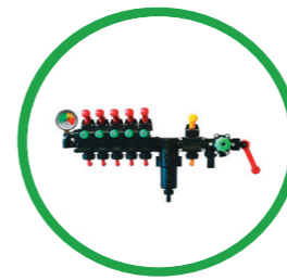
5-ти поточный распределитель постоянного давления
