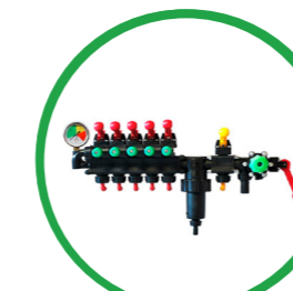
5-ти поточный распределитель постоянного давления
