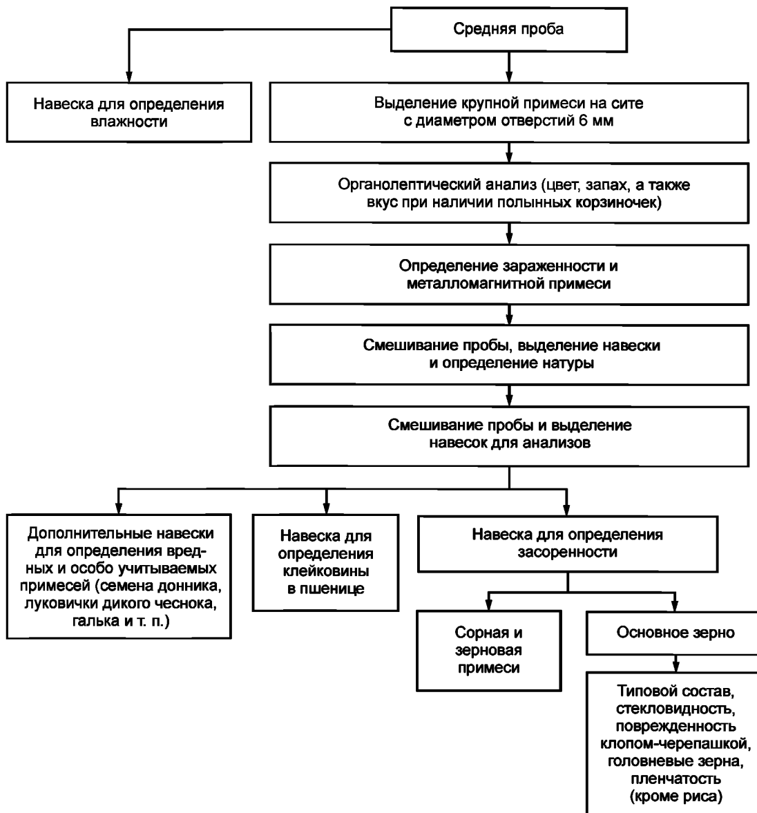
Рисунок 2 — Схема проведения лабораторного анализа средней пробы
